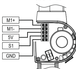
Motore 1 / Motor 1
